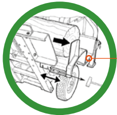
Schnittverstellung mit Auswurfblech für Förderband
