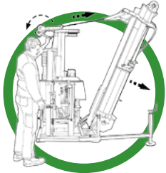
Handwinde zur Ausrichtung des Förderbandes
