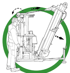
Verricello manuale per il posizionamento del nastro trasportatore
